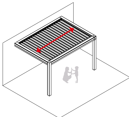
VARIANTE WANDMONTAGE LAMELLEN 90° ZUR WAND
